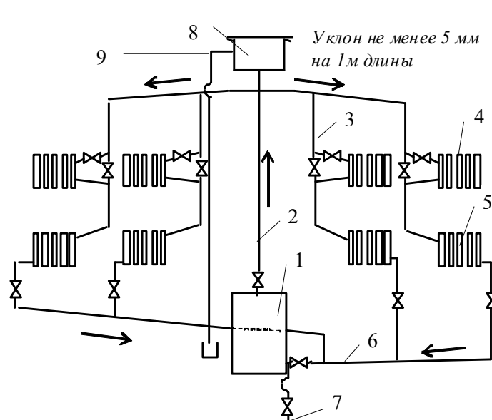
Рисунок 1 - Схема системы отопления
