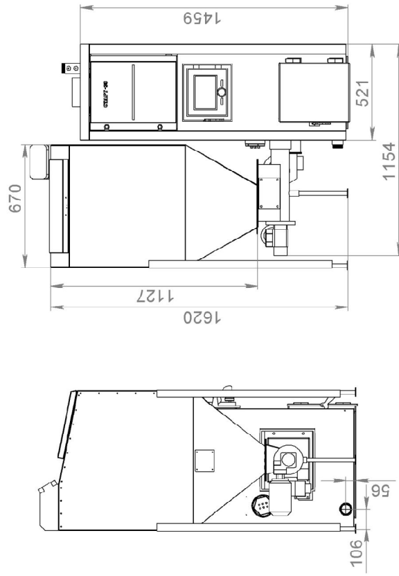
Пеллетный котел "СТАРТ-30-GR-V1", бункер 400 литров
