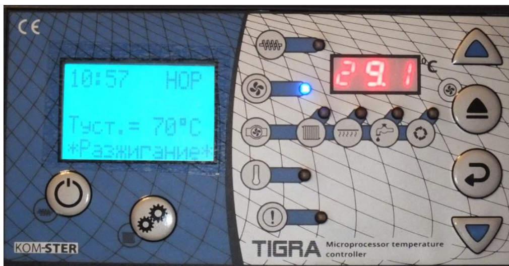
Рисунок 10 – Внешний вид панели управления
